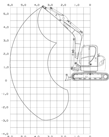
Abb. 1: Hubkrafttabellen EZ80
